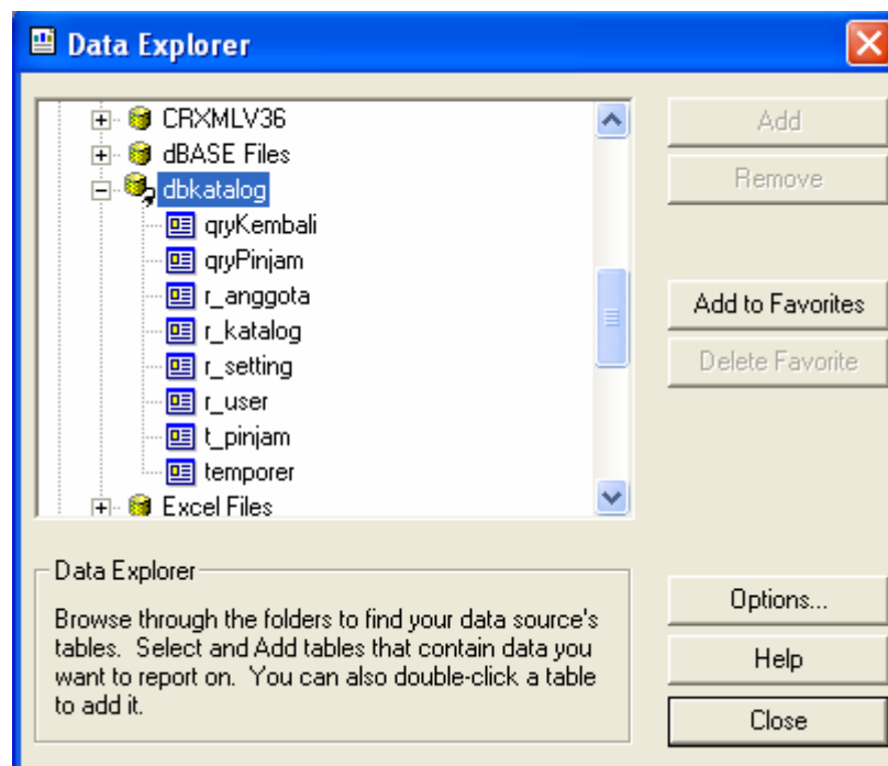
Gambar 4.25 Tampilan DSN
