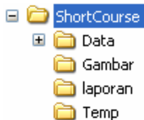
Gambar 4.1 Gambar Direktori
