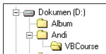
Gambar 1.15 Direktori Kerja
